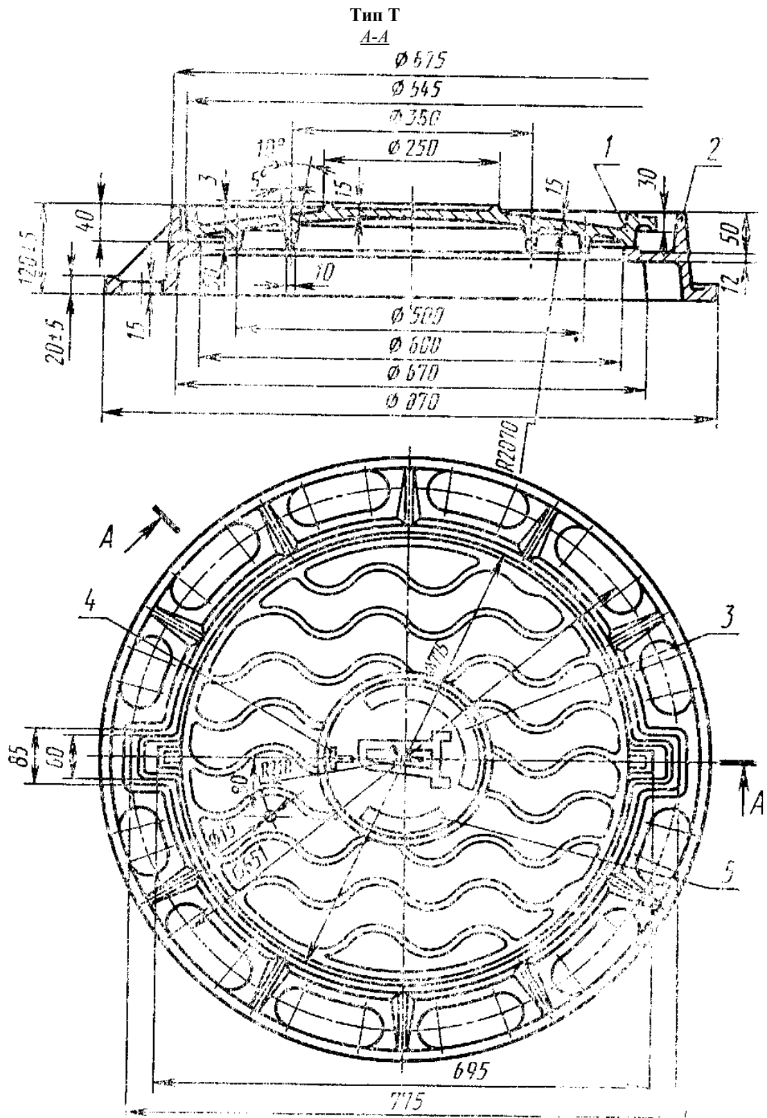
1 - крышка; 2 - корпус; 3 - обозначение настоящего стандарта и год выпуска; 4 - обозначение типа люка; 5 - товарный знак Черт. 2
